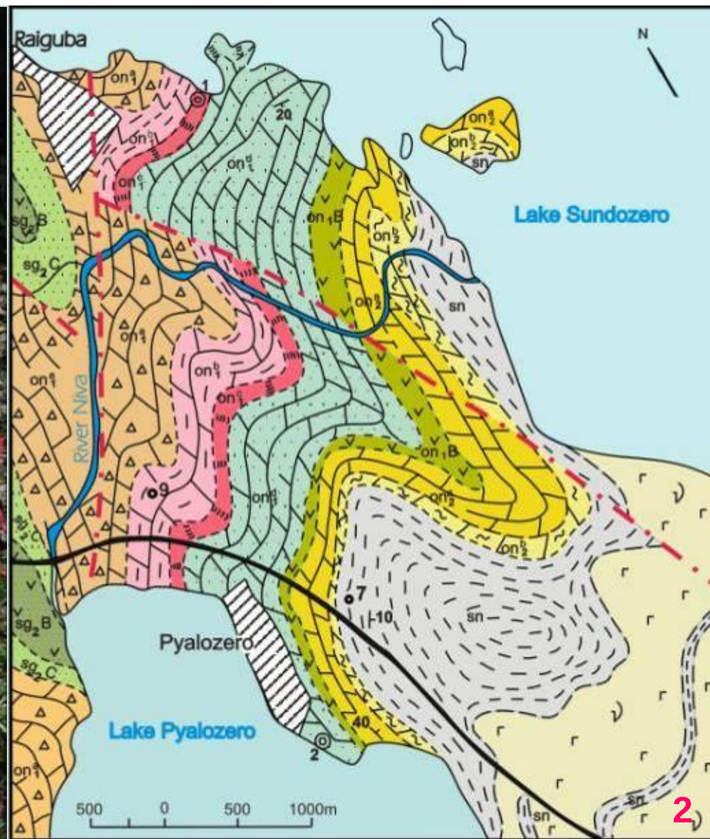
2. Стратотипическая площадь онежского горизонта.
