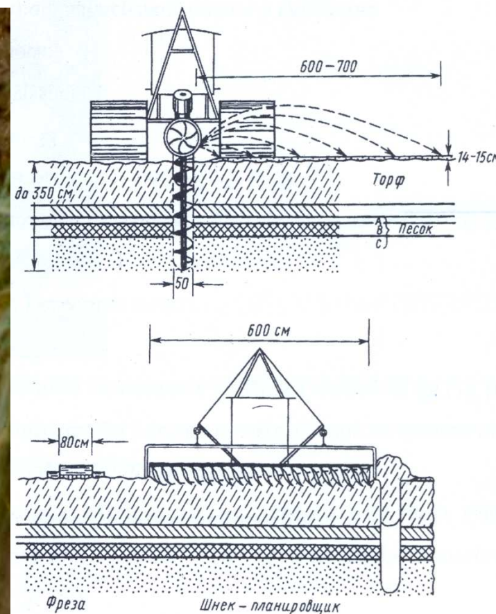
14. Машина для извлечения на поверхность осушенных торфяных почв песка (супеси) и формирования насыпного минерального пахотного горизонта. Планировка и фрезерование поверхности после прохода машины. Римпауская культура земледелия осушенных торфяных почв (К. Готлих, 1980)
