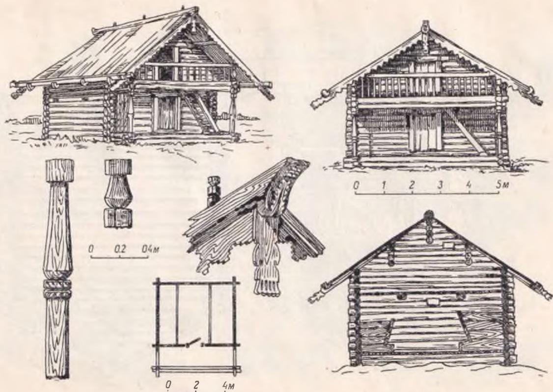
Табл. IX. Амбар дер. Коккойла Прионежского района (в настоящее время находится в Музее архитектуры и этнографии на о. Кизи).
