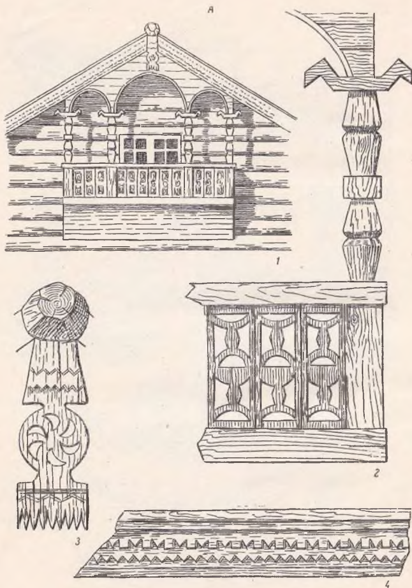
Табл. IV. Архитектурные детали домов Припонежского района.
