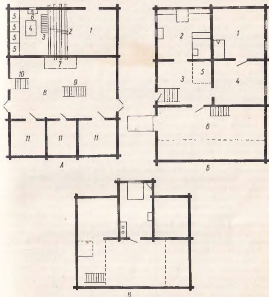
Рис. 27. План дома Н. И. Прокошьева.
