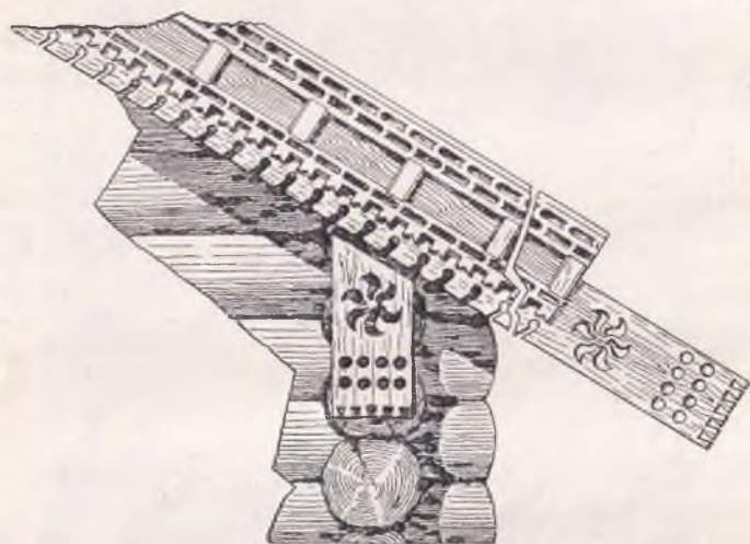
Рис. 18. Фрагмент причелины с «полотепцем».
