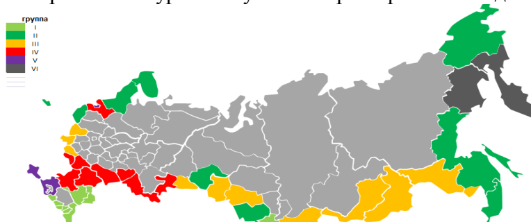
Рисунок 1. Карта-схема пространственного распределения приграничных регионов, относящихся к различным группам типологии по влиянию фактора приграничного положения на развитие региональной туристско-рекреационной системы.
