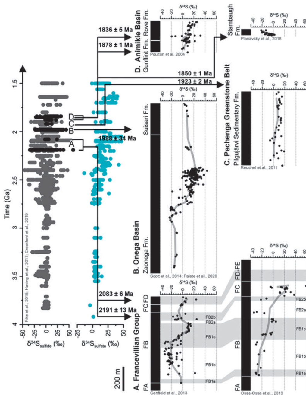
Рис. 14. Изменения значений \delta^{34}S в докембрии с трендами профилей \delta^{34}S из пиритов для разрезов палеобассейнов: Франсвиллиан (2 варианта стратиграфического расчленения), Онежского, Печенгского и Анимики
