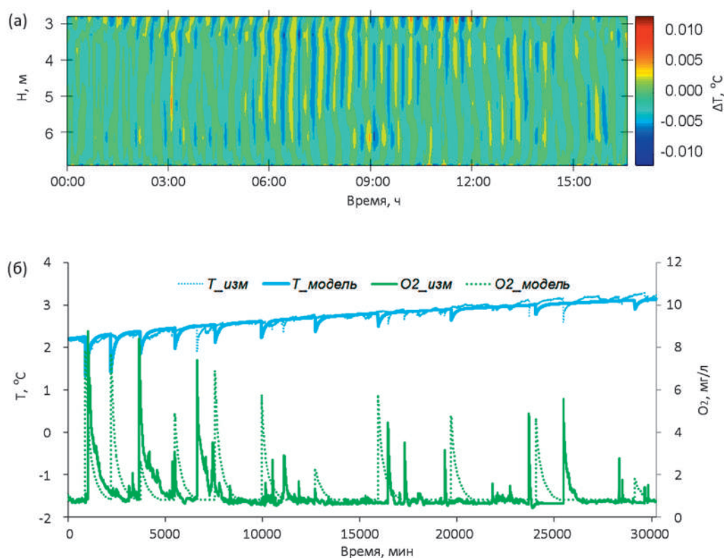
Рис. 7. (а) – проявления внутренних волн в колебаниях температуры водной толщи озера Вендюрского 10 января 2008 г.; (б) – влияние неустойчивости Рэлея-Тэйлора на временную изменчивость температуры и концентрации растворенного кислорода в придонном слое озера Вендюрского, в период с 11 по 31 декабря 2009 г. (время указано в минутах)
