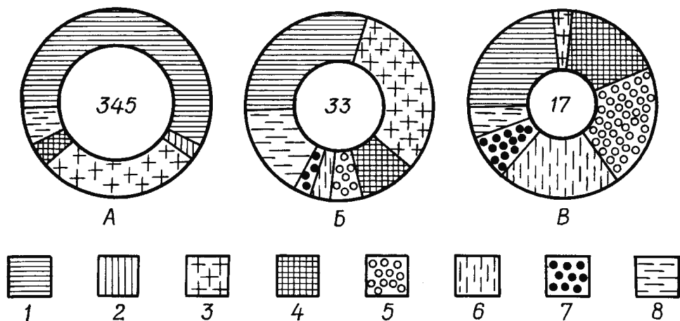
Рис. 8. Влияние контактной обработки глифосатом на видовой состав и массу травянистой растительности: 1 – ве́йник, 2 – луговик, 3 – иван-чай, 4 – ко́стяника, 5 – ландыш, 6 – майник, 7 – седмичник, 8 – разнотравье (цифрами указана воздушно-сухая масса растений, г/м 2 ); А – контроль; Б – 2 кг/га; В – 3 кг/га (по д.в.);
