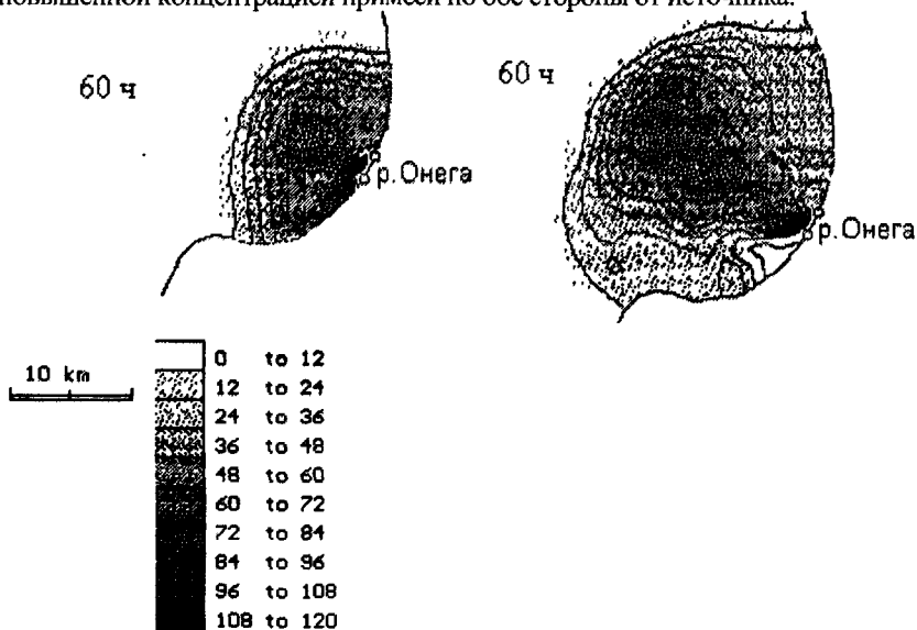
Рис. 2. Распространение примеси в устье р. Онеги при среднегодовом (слева) и максимальном (справа) расходе реки за 60 ч счета.
