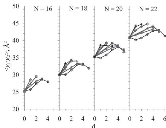
Рис. 5. Зависимости величин средней «площади поперечного сечения» \langle g_1 \cdot g_2 \rangle от количества d двойных связей cis для невозмущенных углеводородных молекул. Условия и обозначения, как на рис. 4
