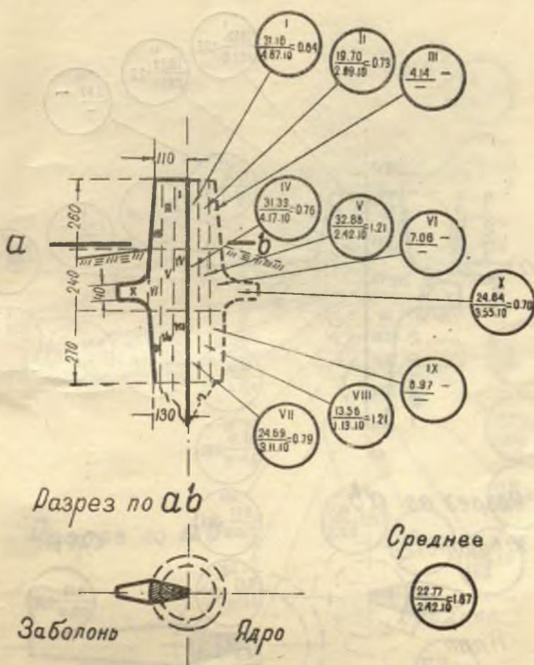
Схема распределения смолы и скипидара в сосновом пне. Образец № 2, взятый в Килевальском р-не, село Ухта. Год рубки 1934. Год корчевки 1949.
