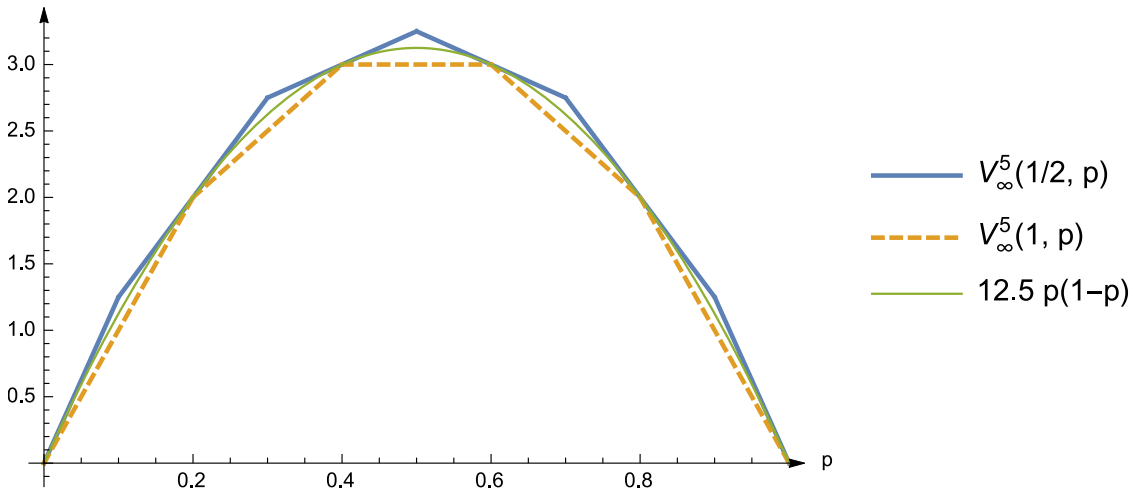
Рисунок 1. Функции V_\infty^m(\beta, p) при \beta = 1/2, 1
