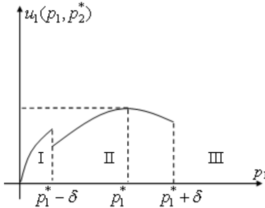
Рисунок 11. Равновесие Хотеллинга
