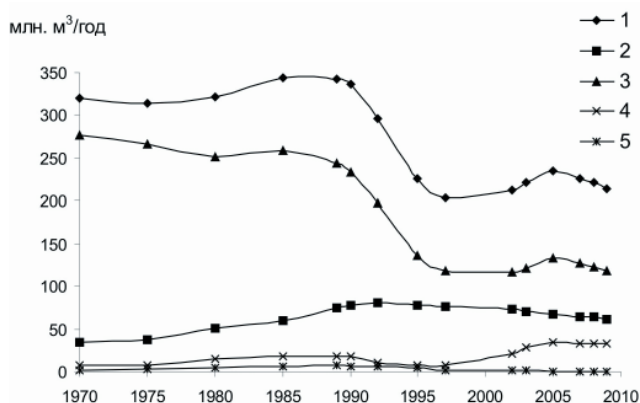
Рис. 2. Динамика водопотребления:
