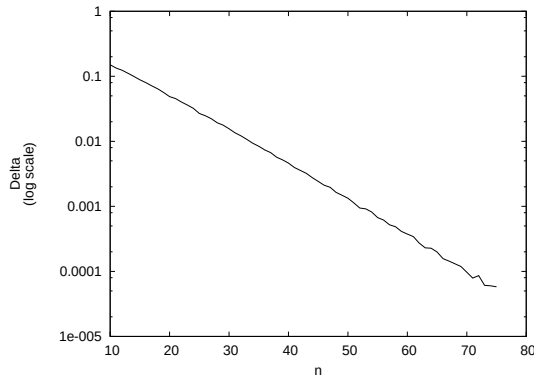
Рис. 4. Зависимость \Delta_n от числа источников
