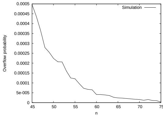
Рис. 3. Зависимость вероятности переполнения \pi_n(1) от количества источников
