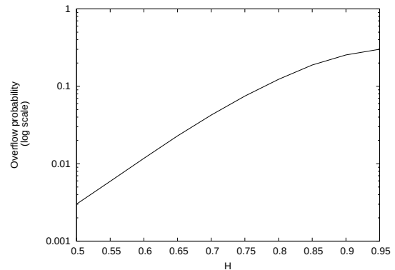
Рис. 5. Зависимость \hat{\pi}_{10}(1) от параметра Херста H
