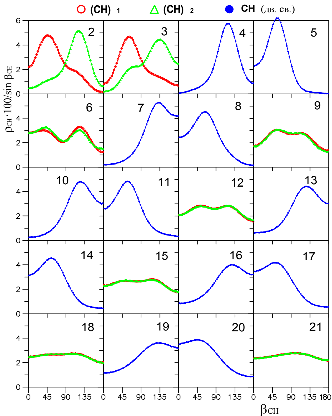
Рис. 6. Гистограммы плотностей вероятности распределения \rho_{CH}(\beta_{CH})/\sin\beta_{CH} по углам \beta_{CH} , образуемым векторами связей C-H цепи 22:6(n-3)cis с нормалью к поверхности гидратированного бислоя 18:0/22:6(n-3)cis ФХ. Цифры 2, 3, ..., 21 означают номера атомов C (номера отвечают рис. 2). Для групп CH_2 гистограммы представлены отдельно для каждой из двух связей C-H
